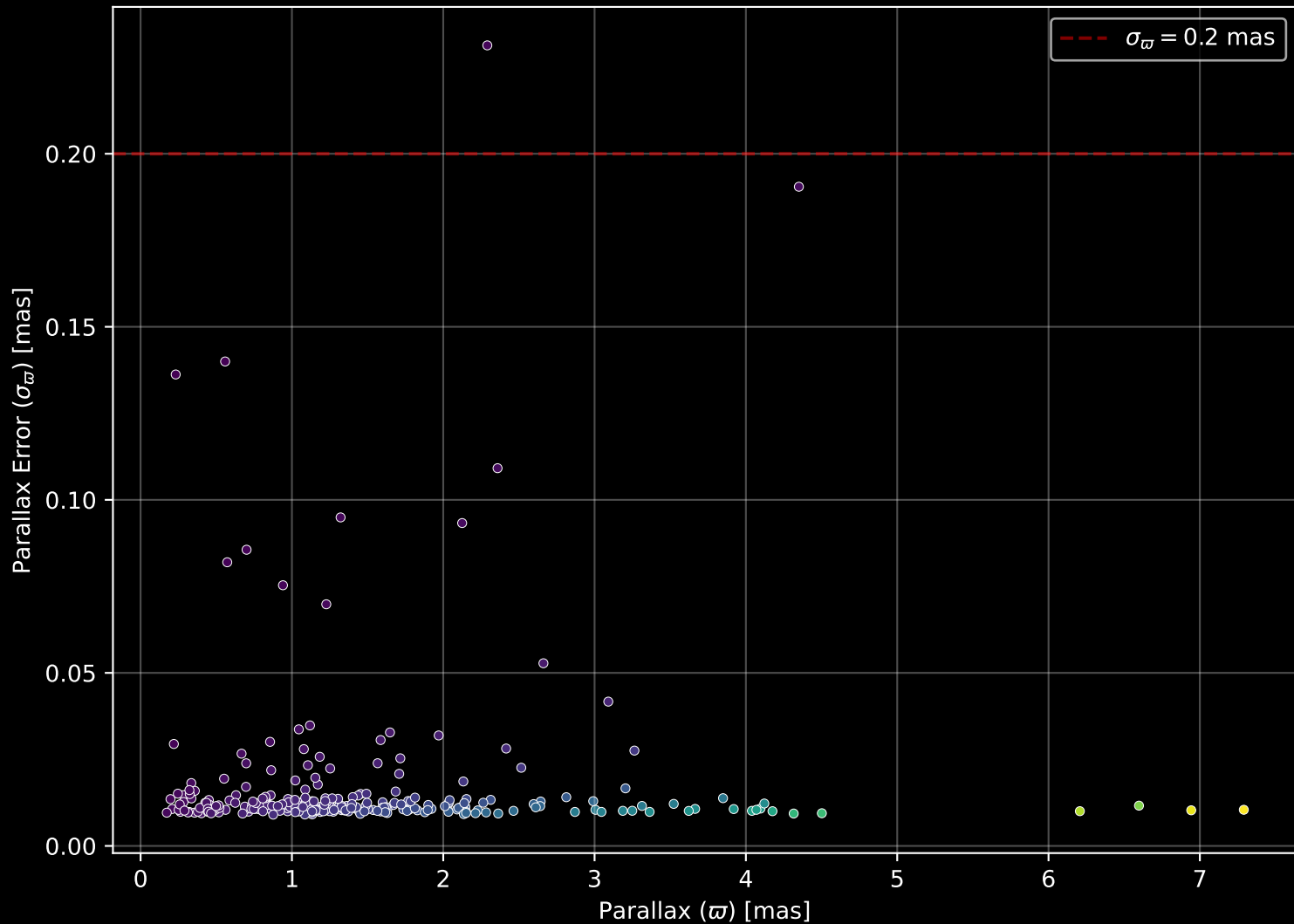
GALAH DR4 Field: [1741] Parallax Quality (n= 277)
