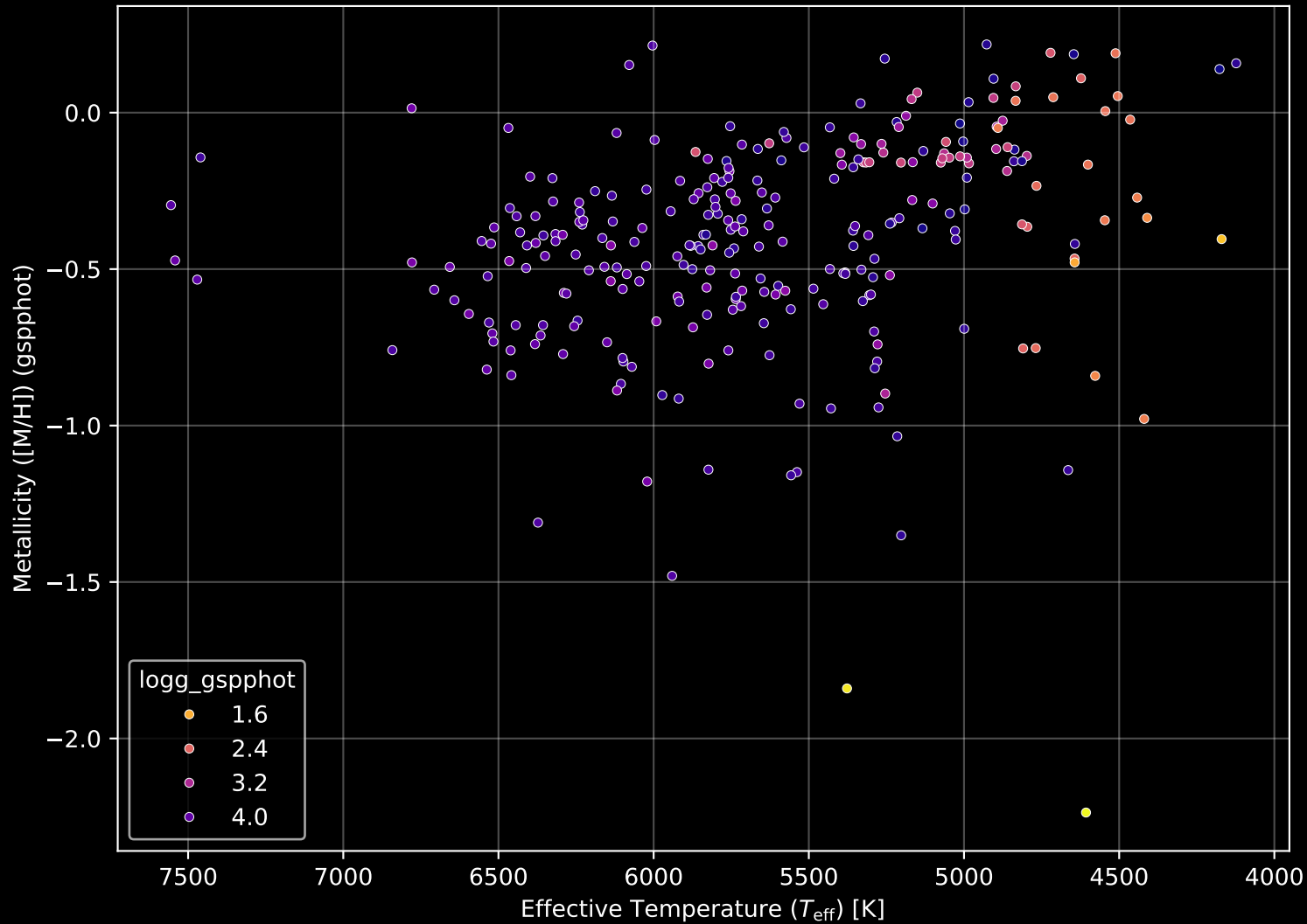
GALAH DR4 Field: [1741] Stellar Population Parameters (n= 277)
