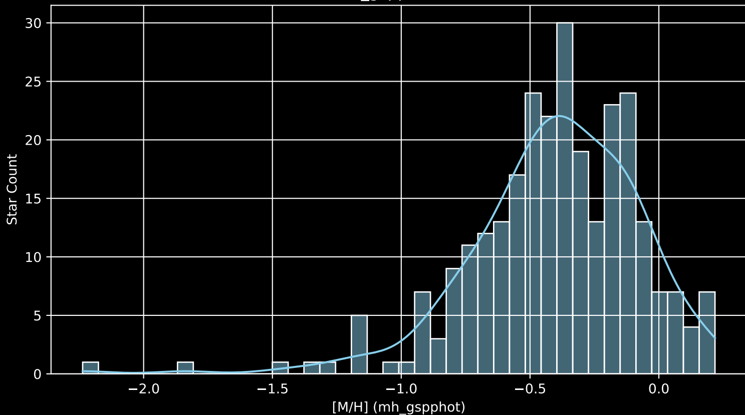
GALAH DR4 Field: [1741] [M/H] (mh_gspphot) (n= 277)
