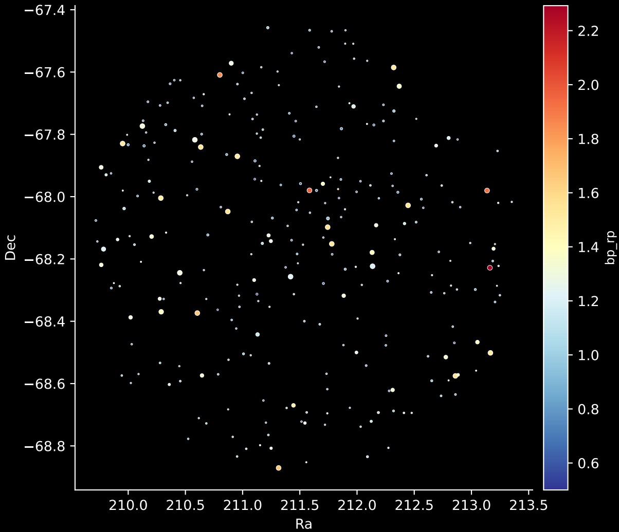
GALAH DR4 Field: [1741] Stars: 277
